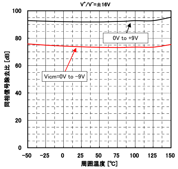
同相信号除去比 対 周囲温度特性例 (同相入力電圧)
