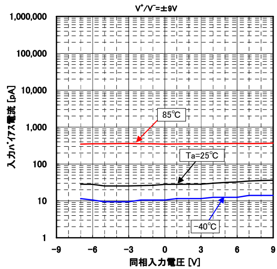
入力バース電流 対 同相入力電圧特性例 (周囲温度)
